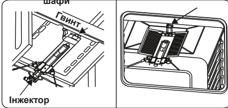
Інжектор
