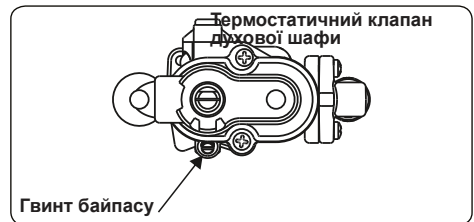
Гвинт байпасу
